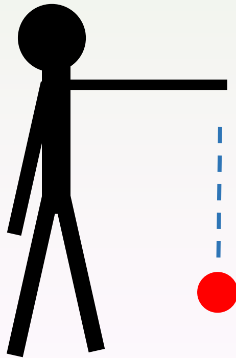
Free Fall
