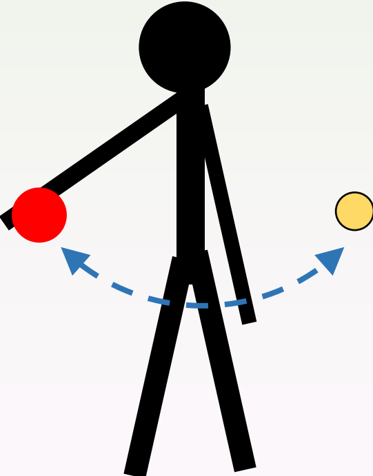
Pendulum
